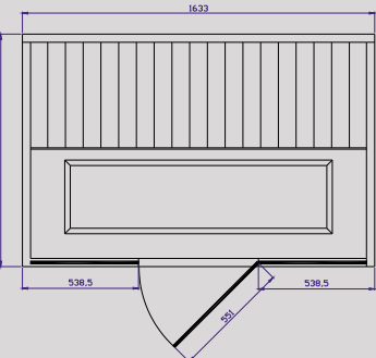
TYLÖSAND T-820 Size: D 1078 x W 1633 mm
