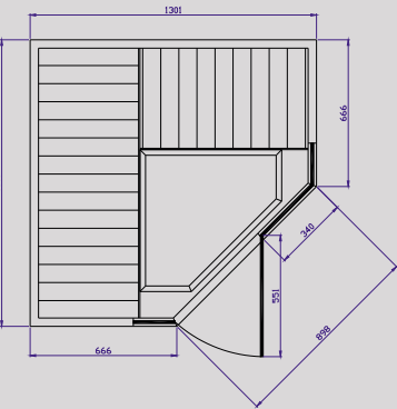
TYLÖSAND T-870 Size: D 1301 x W 1301 mm
